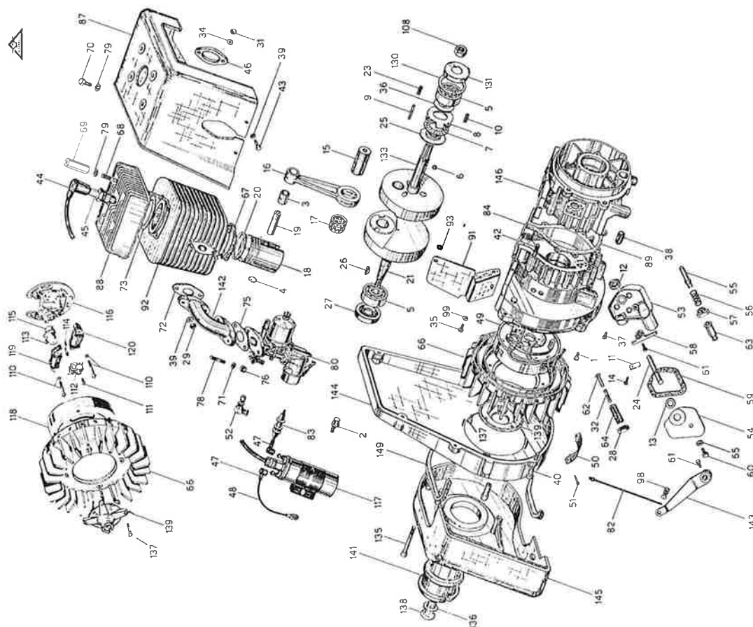
TAV. 9 — MOTORE F.B. MINARELLI I-160 A ROTAZIONE DESTRA
