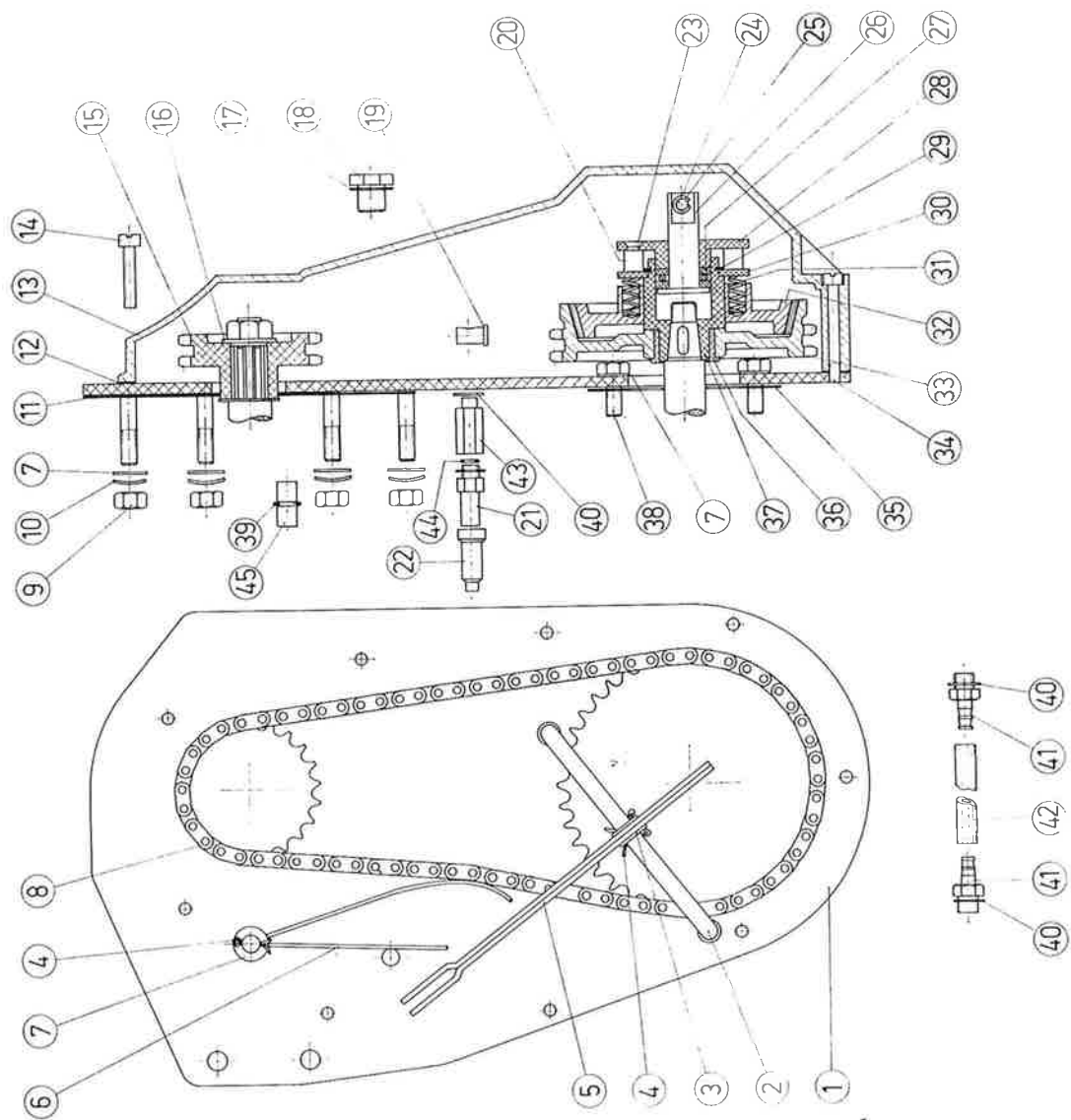
TAV. 11 — GRUPPO FRIZIONE RT 12
