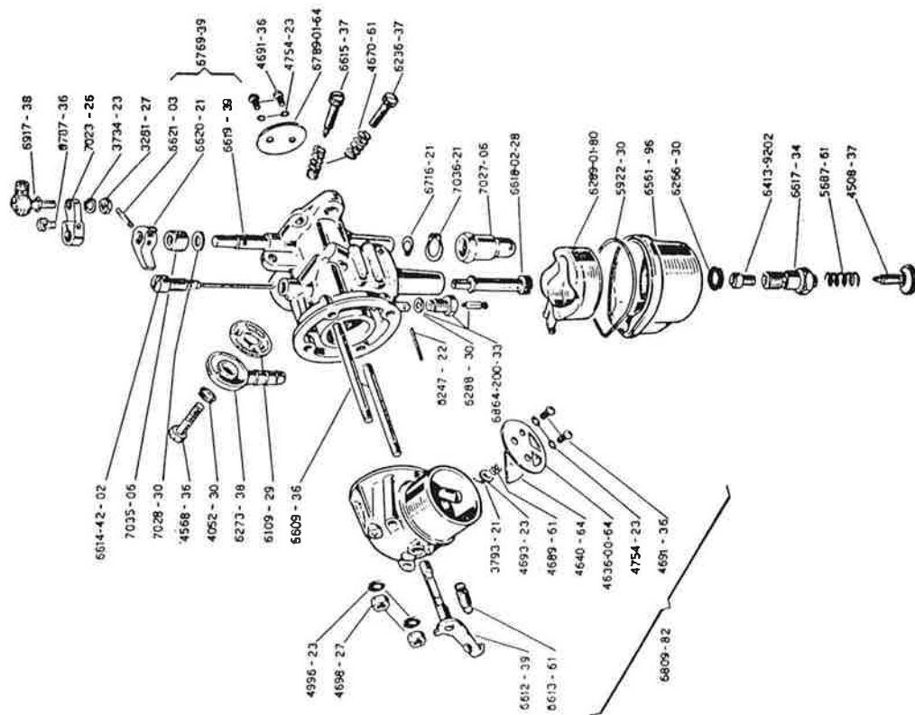
TAV. 10 — CARBURATORE DELLORTO FHE-22-19
