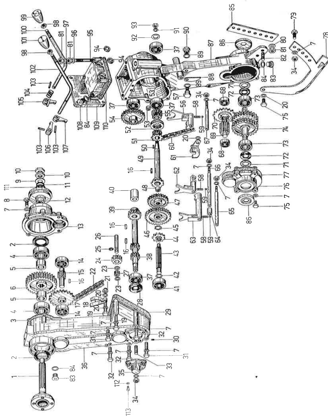
TAV. 5 — GRUPPO TRASMISSIONE RT 10 — RT 12
