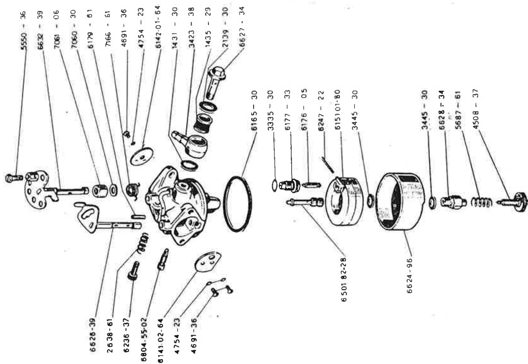
Tav. 5 - Carburatore Dellorto FHC 20-16
